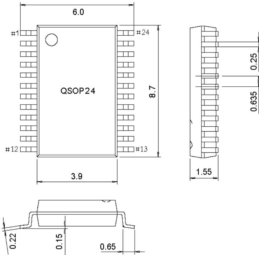
图 4-1 QSOP24 封装
