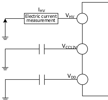
图 3-2-3 CH32M007G8R6 电流消耗测量
