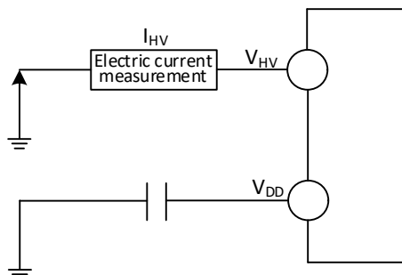
图 3-2-2 CH32M007E8R6 电流消耗测量
