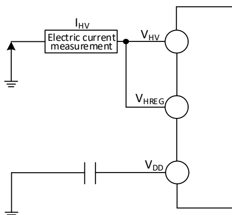
图 3-2-4 CH32M007E8U6 电流消耗测量
